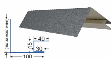
ВІДКОС
