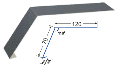
КАПЕЛЬНИК
