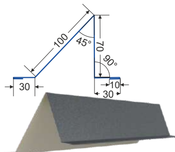
СНІГОЗАТРИМУВАЧ
