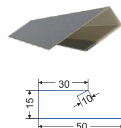
J-ПРОФІЛЬ (СТАРТОВИЙ) (розгортка 10,5 см)
