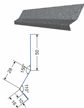
СТАРТОВА ПЛАНКА
