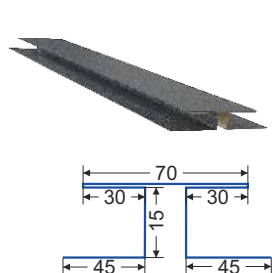
ПЛАНКА СТИКУ (розгортка 25 см)
