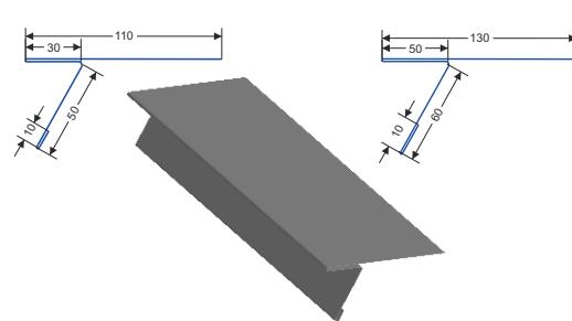
ПРИМИКАЮЧА ПЛАНКА
