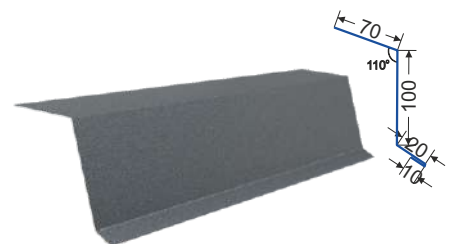
КАРНИЗНА
