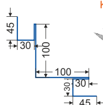
КУТ ВНУТРІШНІЙ (тип 1)
