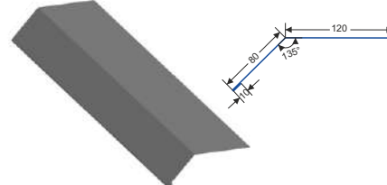
КАПЕЛЬНИК
