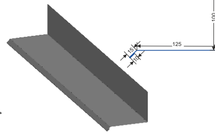
КАПЕЛЬНИК
